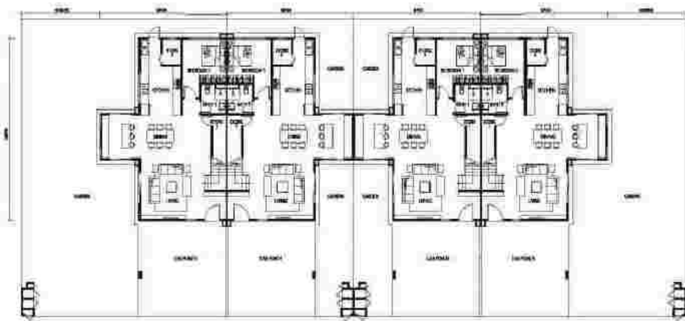
TYPE GH5D3a End
